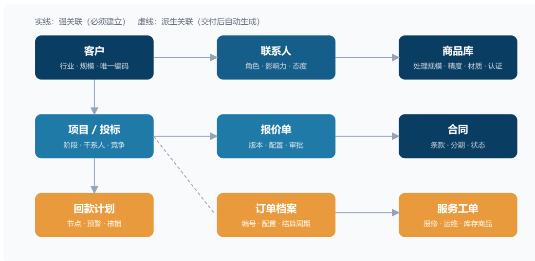
图 4-3 商业贸易行业 CRM 核心数据实体关系示意
