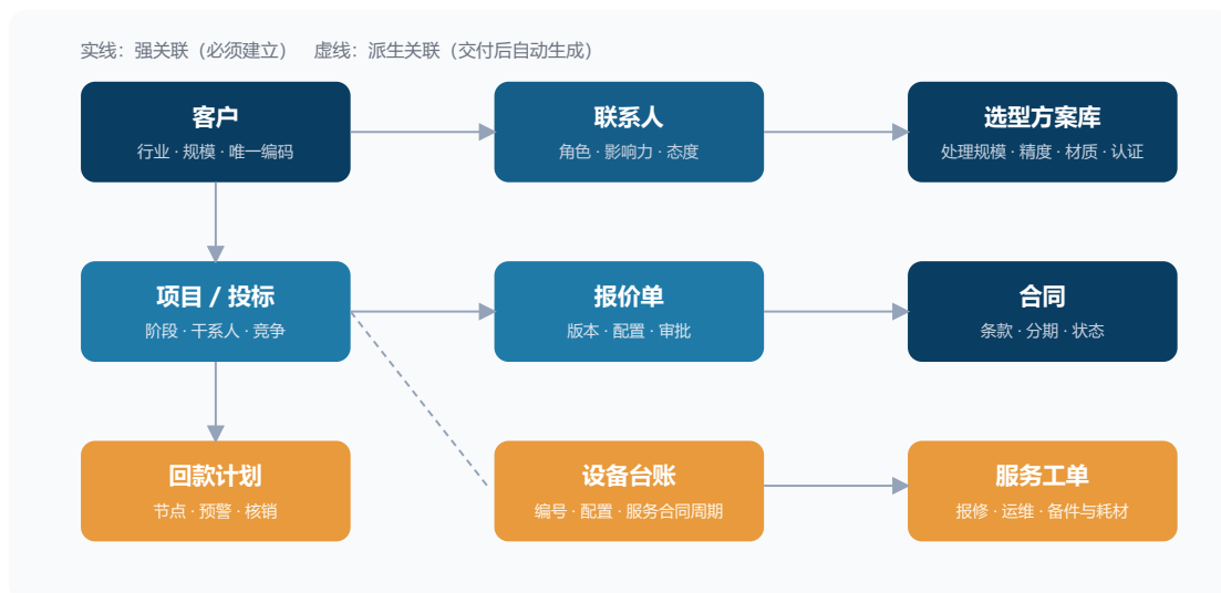
图 4-3 设备销售行业 CRM 核心数据实体关系示意
