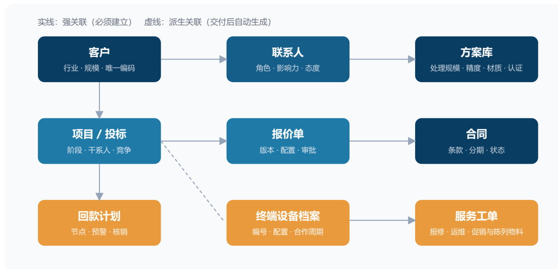
图 4-3 快消行业 CRM 核心数据实体关系示意
