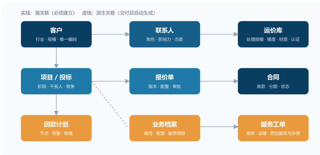
图 4-3 货代行业 CRM 核心数据实体关系示意
