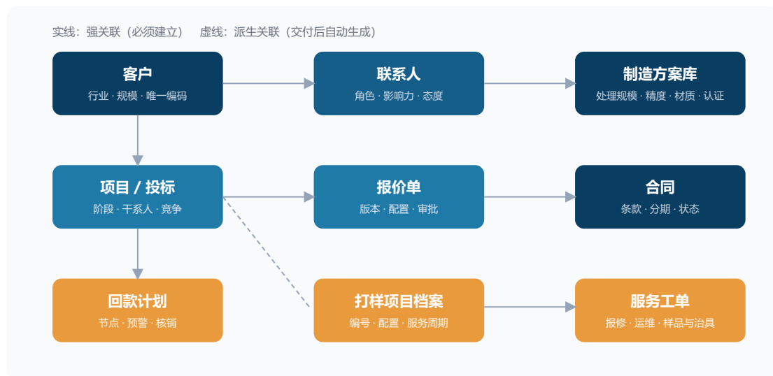
图 4-3 电子行业 CRM 核心数据实体关系示意
