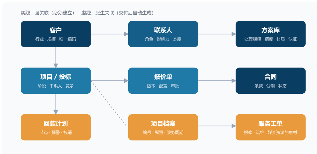
图 4-3 传媒行业 CRM 核心数据实体关系示意
